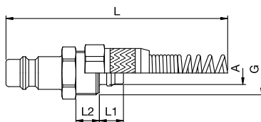
przyłącze do węża z tworzywa ze sprężyną ochronną
