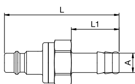
z tłumikiem zwrotnym i tuleją do węża
