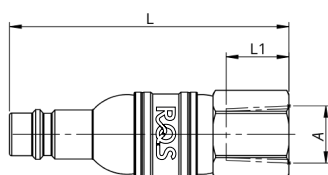
połączenie przegubowe z gwintem wewnętrznym
