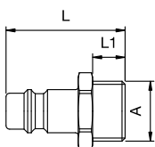
gwint zewnętrzny
