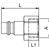
gwint wewnętrzny
